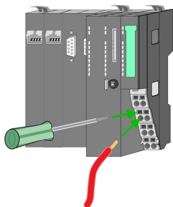
Standard-Verdrahtung
